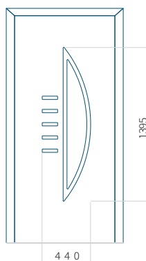
Maximale afmeting van paneel
